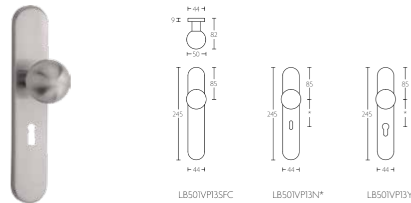
LB501VP13 meterkastknop vast op schild | cabinet knob fixed on plate
